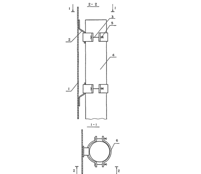
1 - щит знака; 2 - скоба знака; 3 - болт крепления хомута; 4 - опора крепления; 5 - гайка крепления хомута; 6 - хомут крепления
