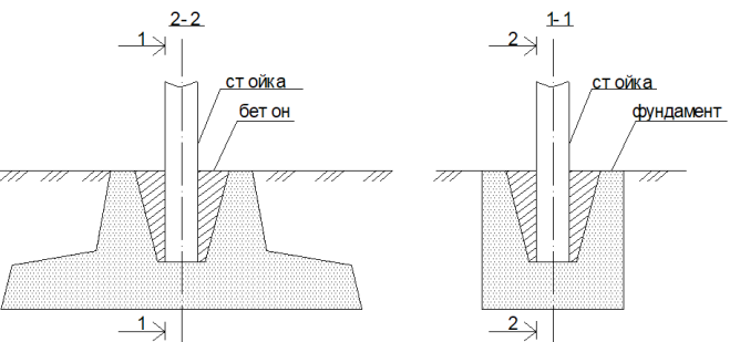
Рис. 2 Крепление щита знаков на опоре типа СКМ.
